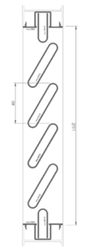
SECCIÓN LAMA FIJA
