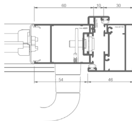
MARCO Y HOJA LATERAL CON CERRADURA
